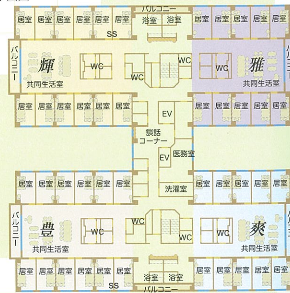
2階平面図
