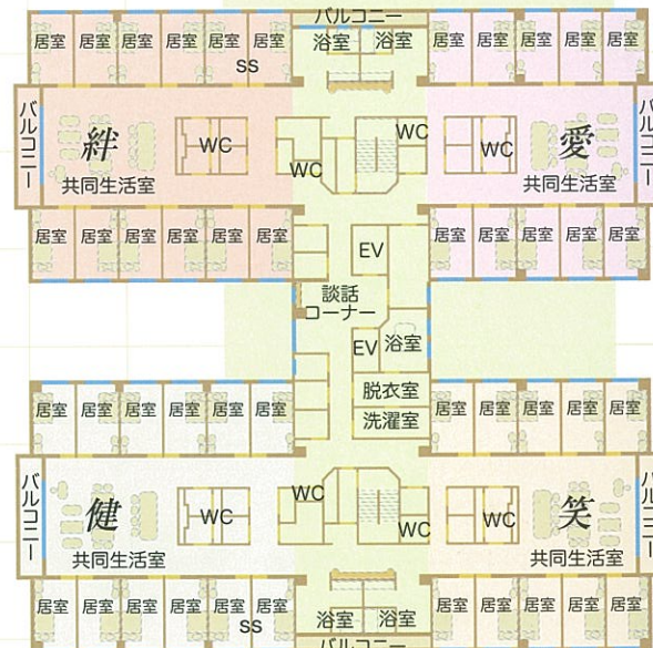
3階平面図
