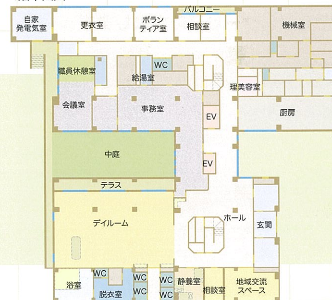
1階平面図
